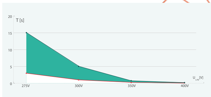
Curva de tensión / tiempo según normativa UNE-EN-50550
