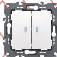
S20.106.XX - Interruptor doble luminoso S20.123.XX - Conmutador doble luminoso
