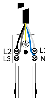
CONECTOR INICIAL VISTA SUPERIOR NEUTRO DERECHA TRCK-009/023
