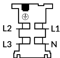
CONECTOR INICIAL VISTA FRONTAL NEUTRO DERECHA TRCK-009/023
