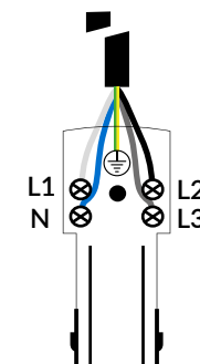
CONECTOR INICIAL VISTA SUPERIOR NEUTRO IZQUIERDA TRCK-038/037
