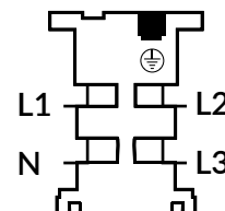
CONECTOR INICIAL VISTA FRONTAL NEUTRO IZQUIERDA TRCK-038/037
