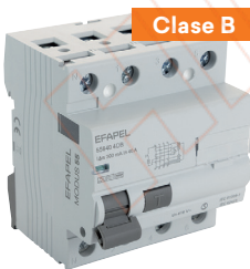
interruptores diferenciales
